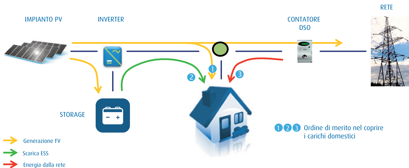
Schema 2: soluzione RESS 1 per impianto FV nuovo 2
